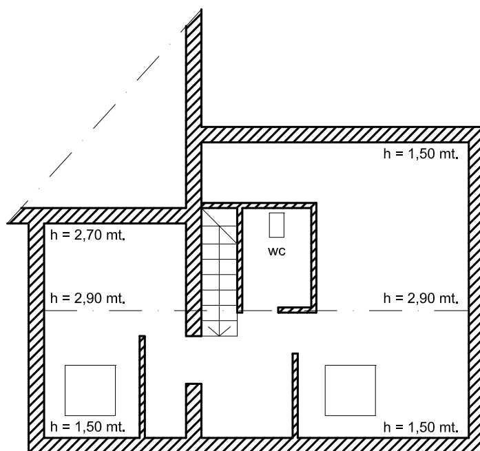
PIANTA PIANO SOTTOTETTO
